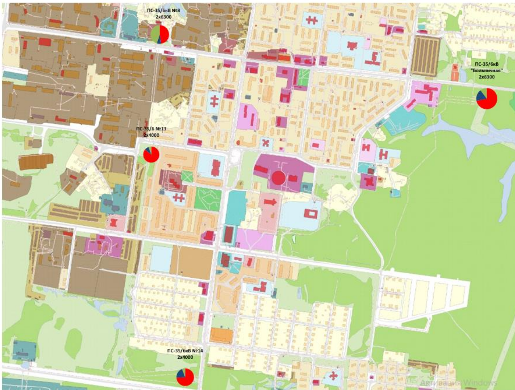
PC-35/6кВ №8 2x6300
