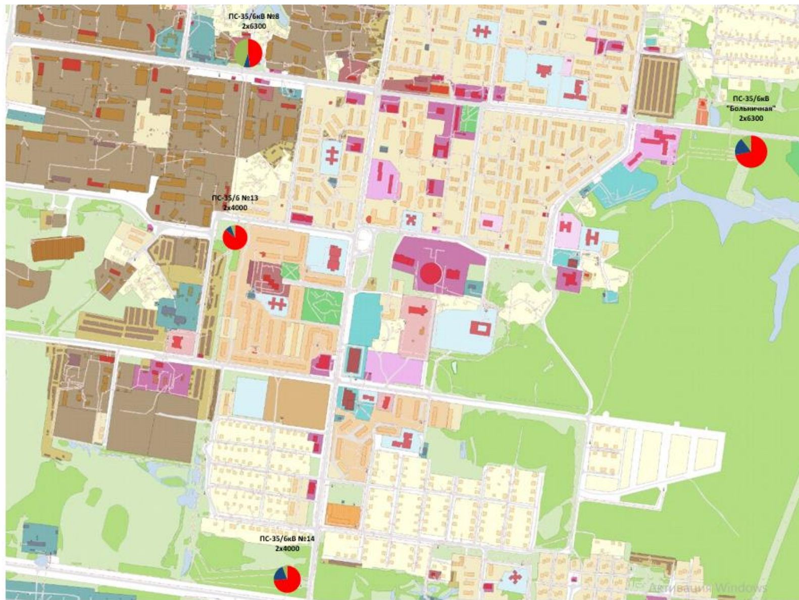
ПС-35/6кВ №8 2х6300
